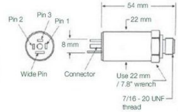
DIN EN 175301-803 connector
